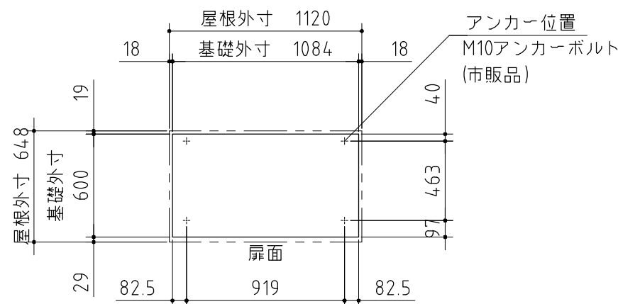
ベタ基礎図
